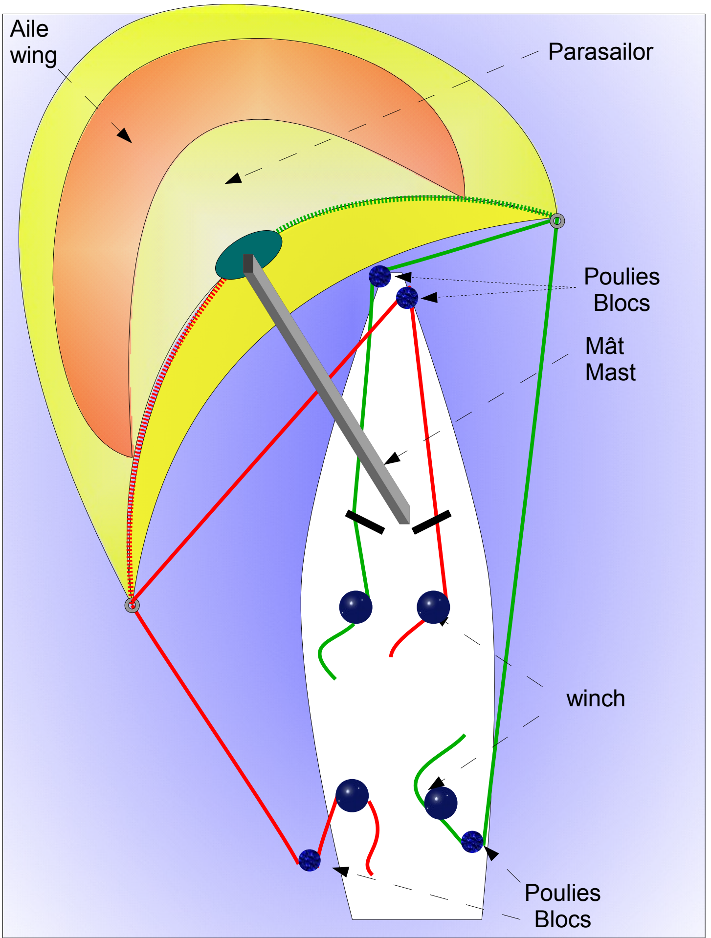
Configuration au portant (down wind)
